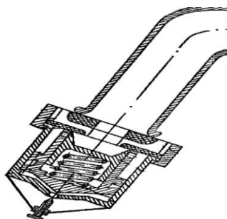
Рис. 2. Распылитель опрыскивателя
